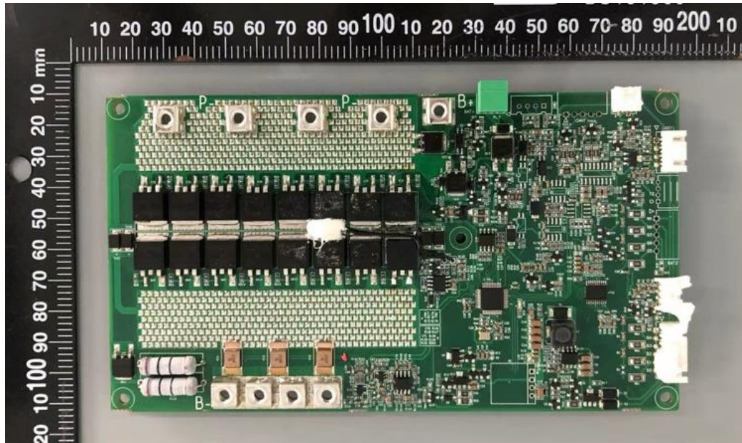
BMS PCBA 1
