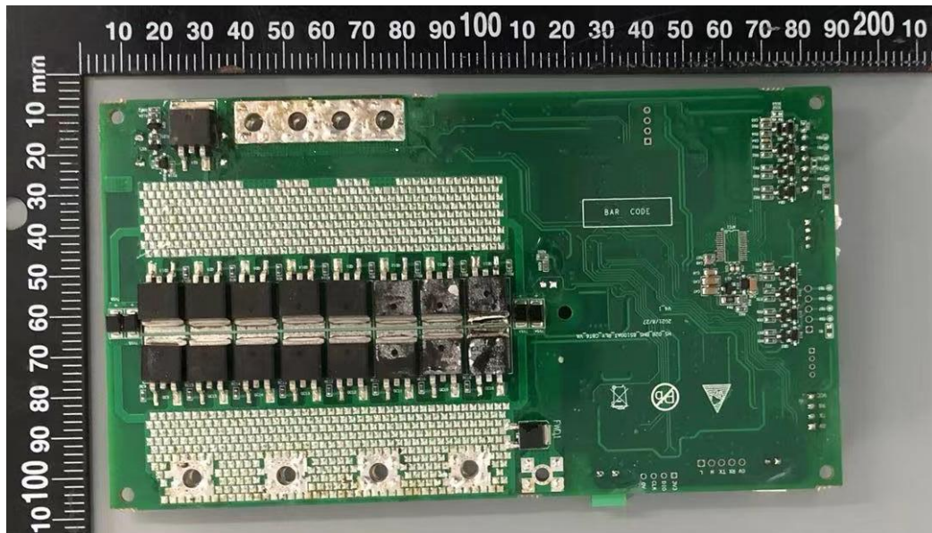
BMS PCBA 2
